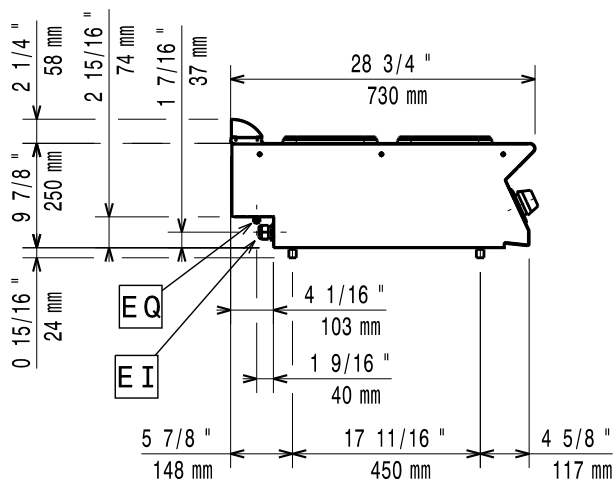
Oldalnézet
